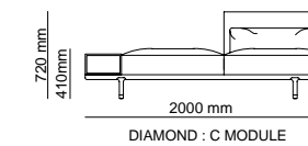
2000 mm DIAMOND : C MODULE
