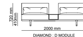
2000 mm DIAMOND : D MODULE
