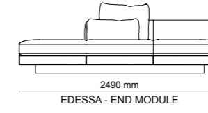
2490 mm EDESSA - END MODULE
